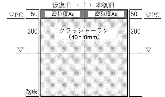
(10)新々田区画整理事業 車道舗装構成（基層無し路線）
