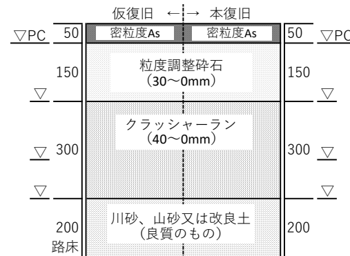
(8)新木駅南側土地区画整理事業 幅員9～12m区画道路舗装構成
