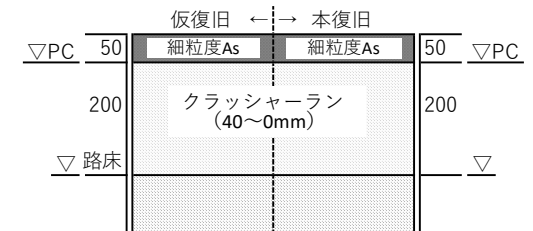
(7)中峠区画整理事業 幅員 9 m 歩道部舗装構成 (車両乗り入れ部)
