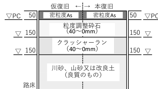
(8)新木駅南側土地区画整理事業 幅員9～12m区画道路舗装構成
