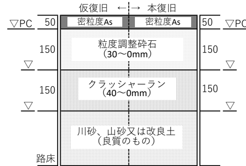
(6)青山区画整理事業 幅員4～6m舗装構成
