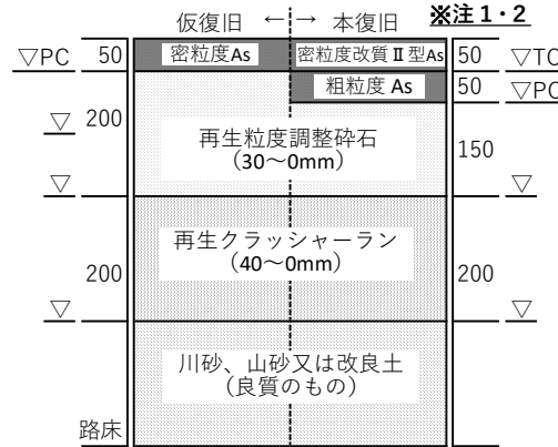
B 型 二層中級舗装
