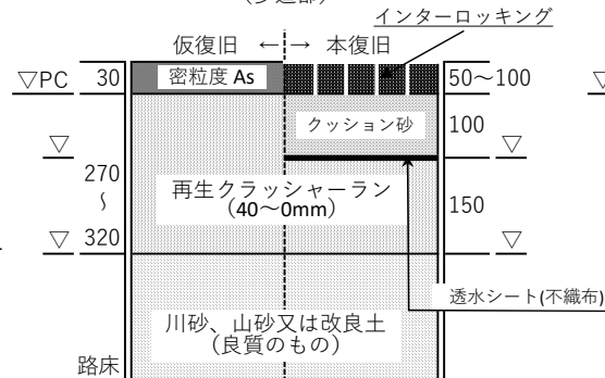
インターロッキング舗装
