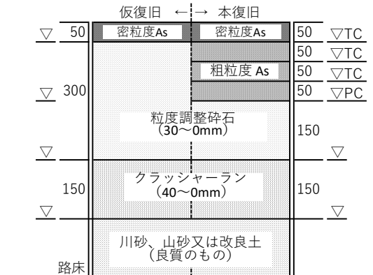
(5)柴崎土地区画整理事業 幅員 1 2 m 舗装構成
