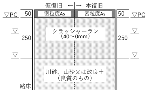
(7)中峠区画整理事業 幅員 5 ～ 8 m舗装構成
