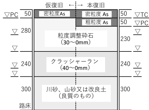
(4)高野山宮脇土地区画整理事業 歩行者専用道舗装構成
