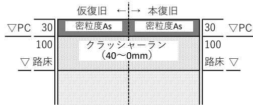
(10)新々田区画整理事業 歩道舗装構成
