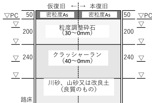
(8)新木駅南側土地区画整理事業 都市計画道路3・5・23号線 幅員16m区画道路舗装構成
