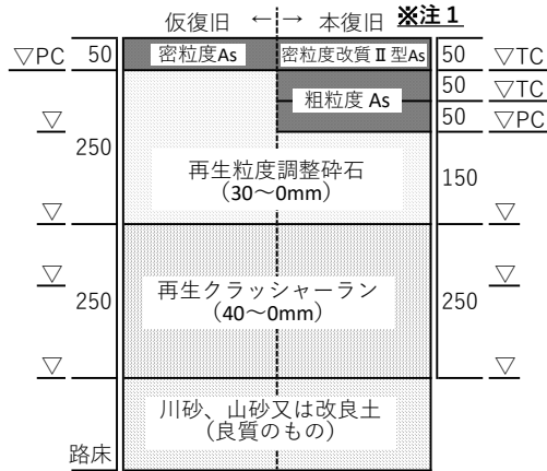
A 型 三層アスファルト舗装
