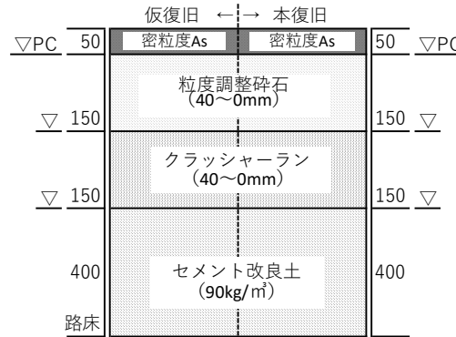
(9)布佐平和台開発事業・布佐西町区画整理事業 幅員 5 ～ 9 m 舗装構成（布佐西町は4～9m）
