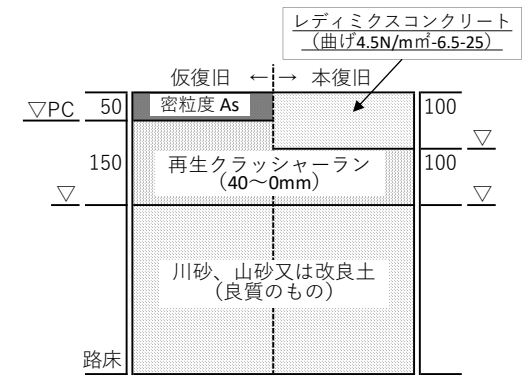
D 型 コンクリート舗装
