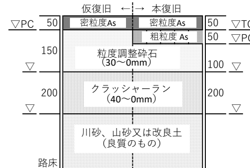
(5)柴崎土地区画整理事業 幅員 8 ~ 9 m 舗装構成
