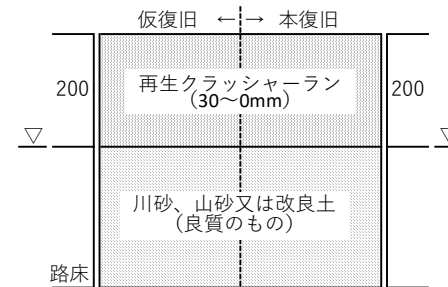
F 型 砂利道
