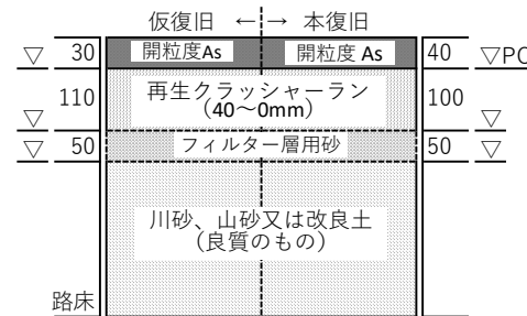
E-Ⅱ 型 歩道透水性舗装
