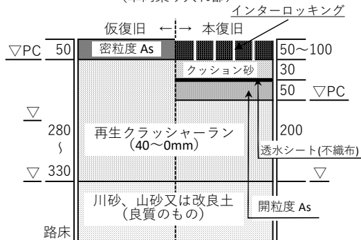
インターロッキング舗装
