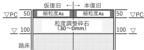
(6)青山区画整理事業 一般歩道舗装構成
