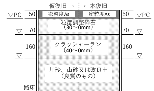
(8)新木駅南側土地区画整理事業 幅員 6 m 区画道路舗装構成
