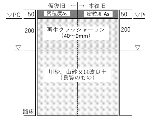
C 型 一層簡易舗装
