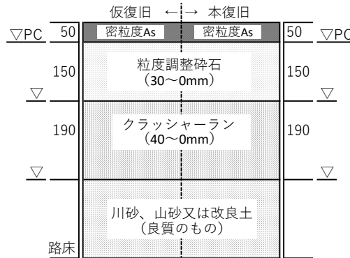
(5)柴崎土地区画整理事業 幅員 4 ~ 6 m 舗装構成
