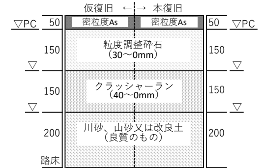
(6) 青山区画整理事業 幅員 12 m 舗装構成
