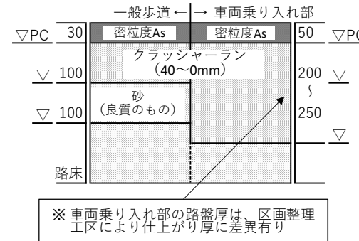
(3)高野山まちづくり区画整理事業 歩道舗装構成
