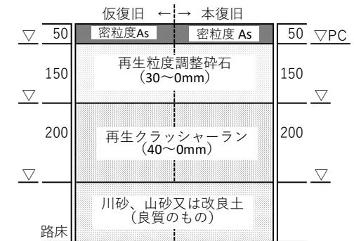
開発行為による道路舗装
