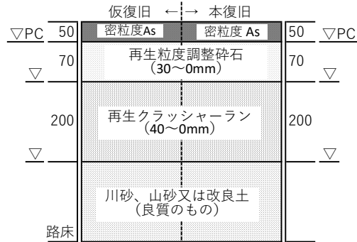
(2)我孫子駅前(北口)区画整理事業 幅員 1 7 m 舗装構成
