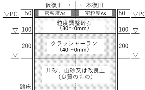
(5)柴崎土地区画整理事業 幅員 4 ~ 6 m 舗装構成
