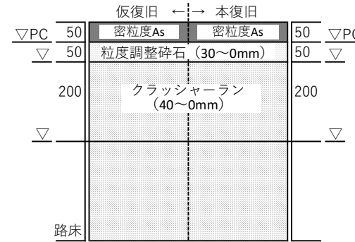
(10)新々田区画整理事業 車道舗装構成（基層有り路線）
