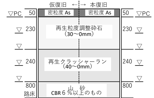
(4)高野山宮脇土地区画整理事業 車道舗装構成
