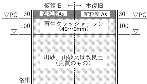
E 型 歩道舗装
