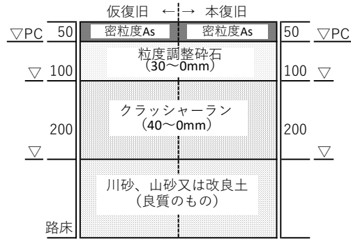
(8)新木駅南側土地区画整理事業 幅員 6 m 街路標準舗装構成
