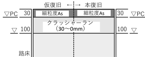
(4)高野山宮脇土地区画整理事業 歩行者専用道舗装構成
