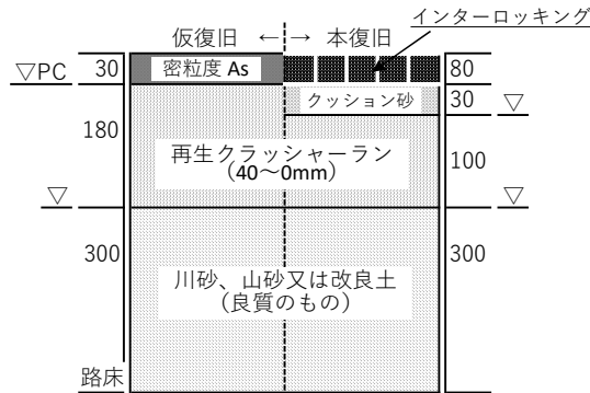
(3)高野山まちづくり区画整理事業 車道舗装構成
