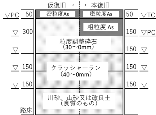
(5)柴崎土地区画整理事業 幅員 16 m舗装構成
