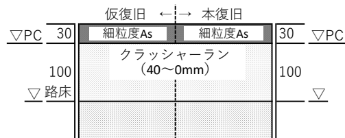
(7)中峠区画整理事業 幅員 9 m 歩道部舗装構成（一般歩道部）
